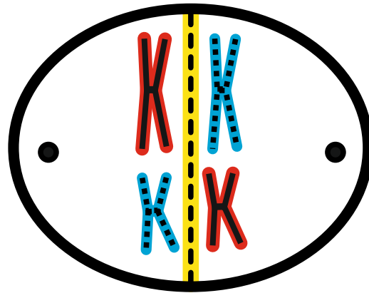
Métaphase 1
