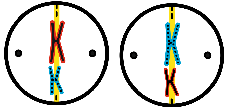
Métaphase 2
