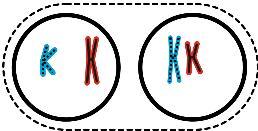
Télophase 1
