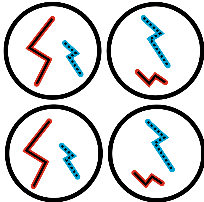
Télophase 2
